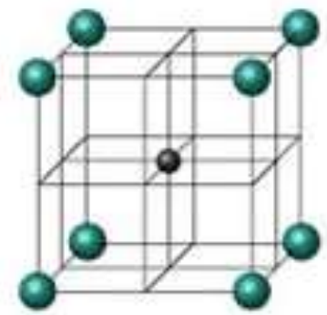
CsCl
